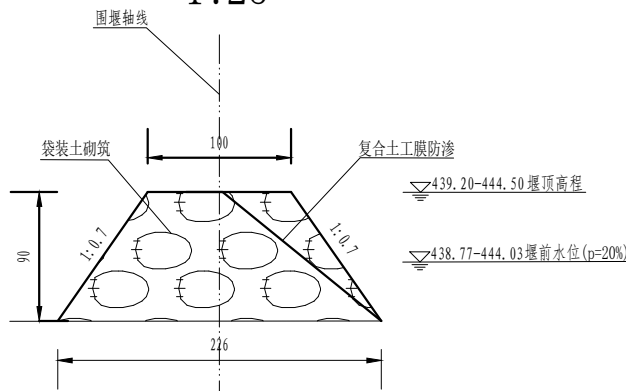
导流围堰典型断面图
