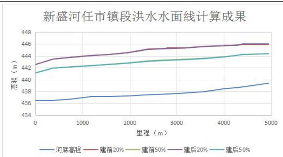
图 2-3 新盛河任市镇段堤防洪水水面计算成果图
