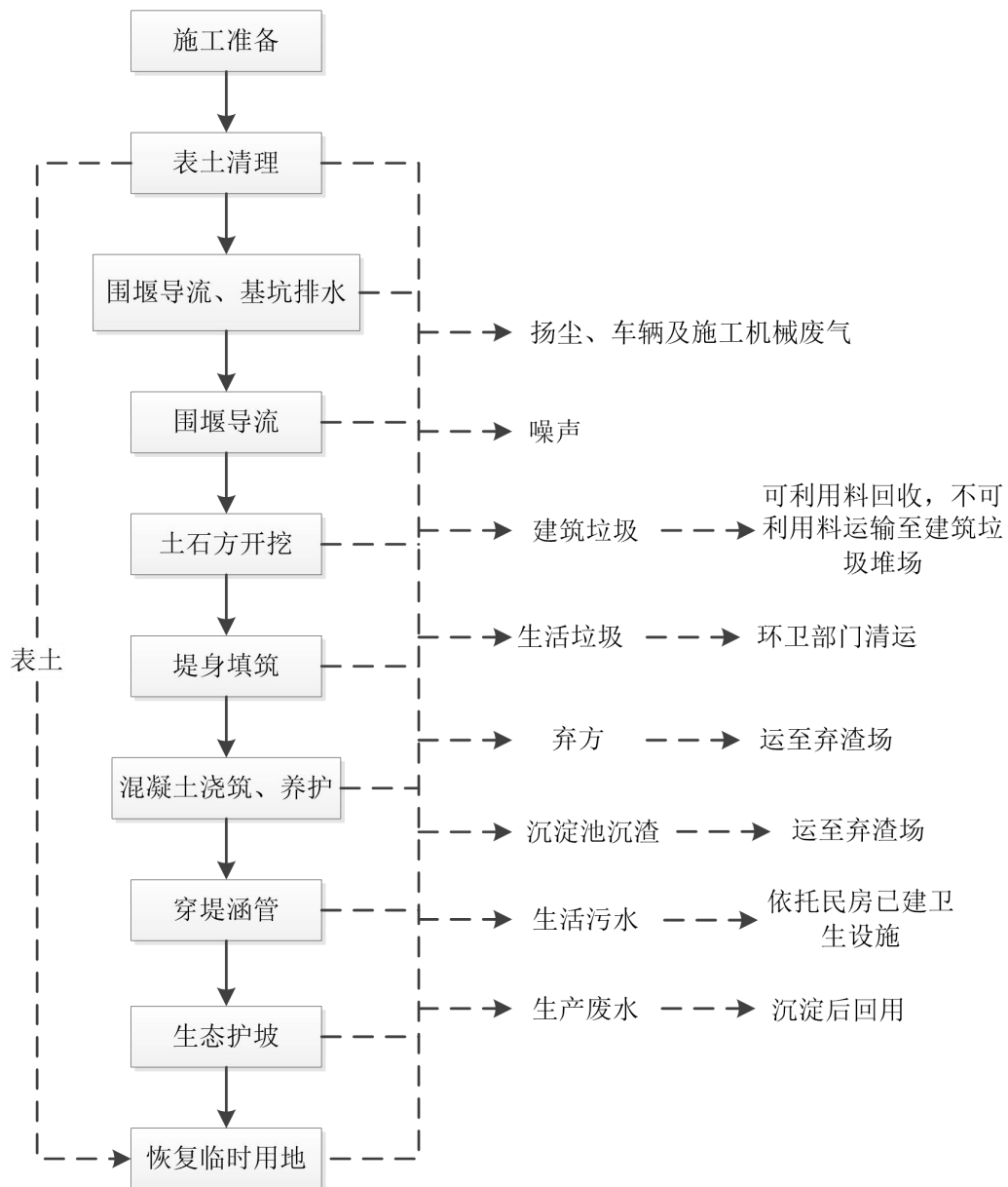
图 2-4 项目施工工艺流程及污染环境图
