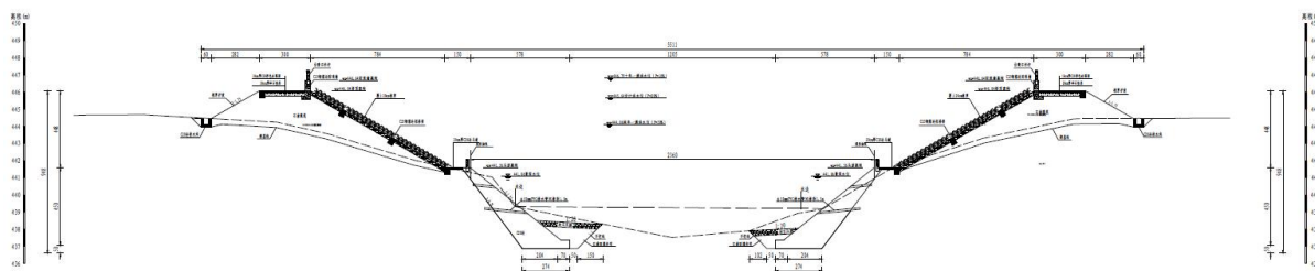
图 2-1 项目堤型断面图
