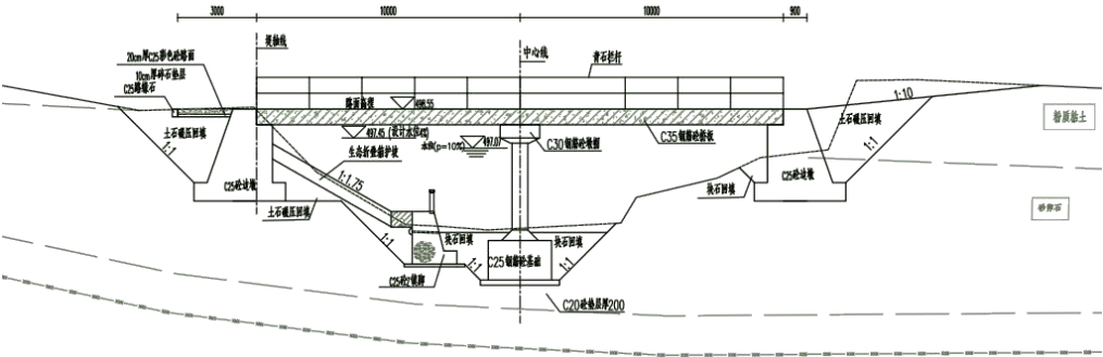
图 2-5 LYL0+903.05 人行桥结构断面图
