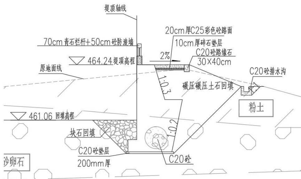
图 2-16 方案四典型断面图
