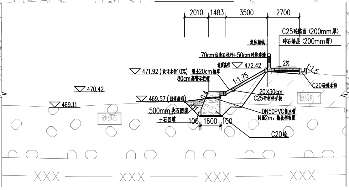
堤岸型式典型断面图
