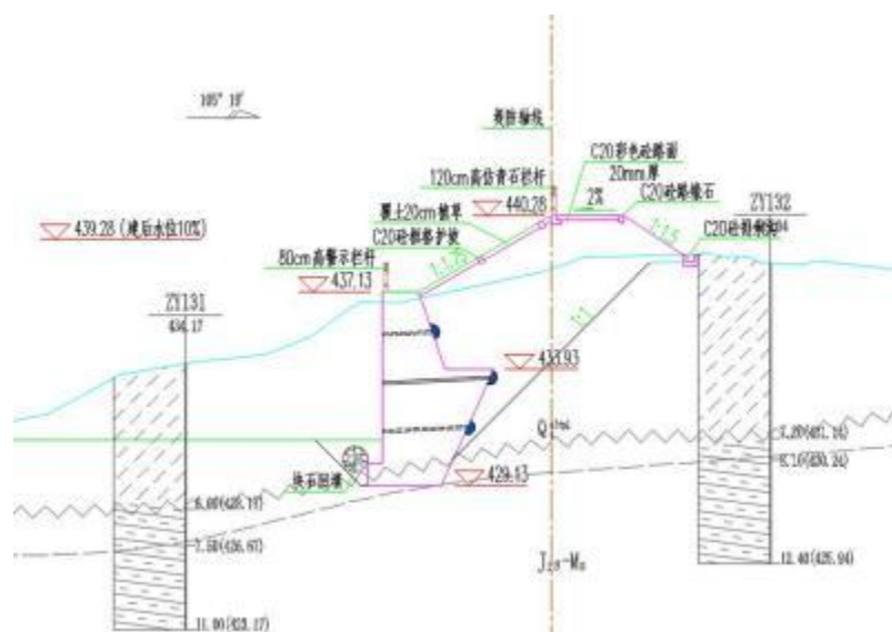
图 2-13 方案一典型断面图
