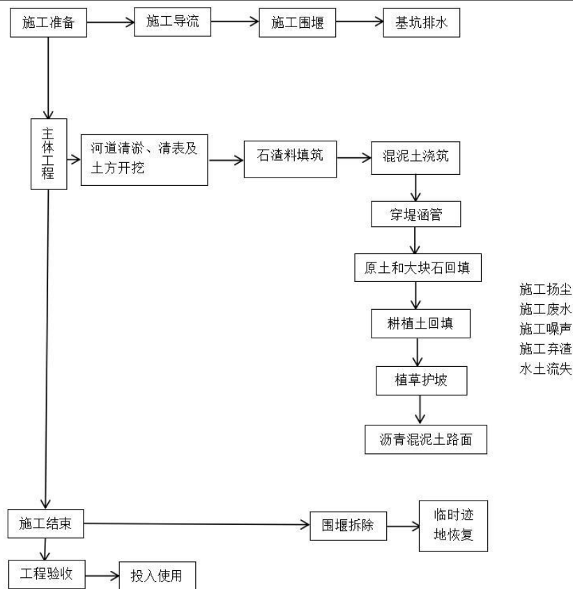
图 2-1 项目施工工艺流程及产污环节图
