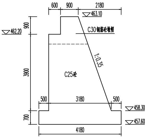
边墩断面图 1:100
