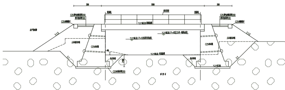
图 2-6 XR1+459.33 人行桥结构断面图
