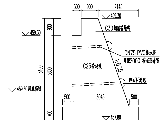
边墩断面图 1:100
