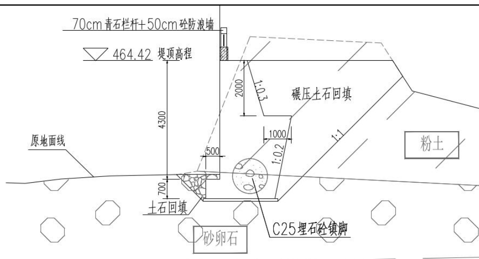
图 2-4 直立式挡墙结构断面图
