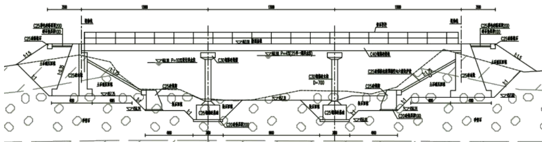
图 2-7 X1+544.61 人行桥结构断面图
