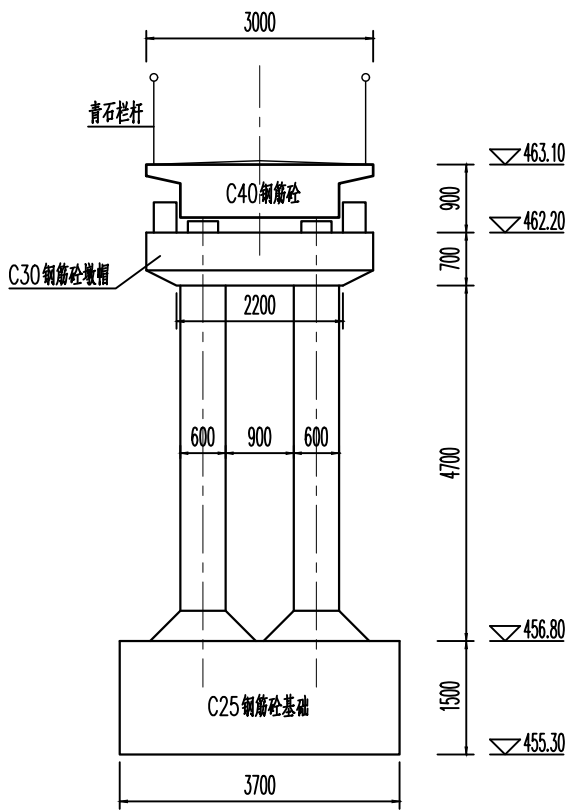
中墩立面图 1:100
