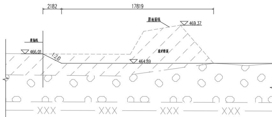
图 2-8 河道清淤典型断面图
