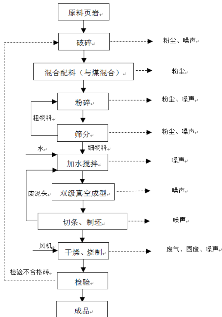
图 2-2 项目生产工艺流程及产污环节图
