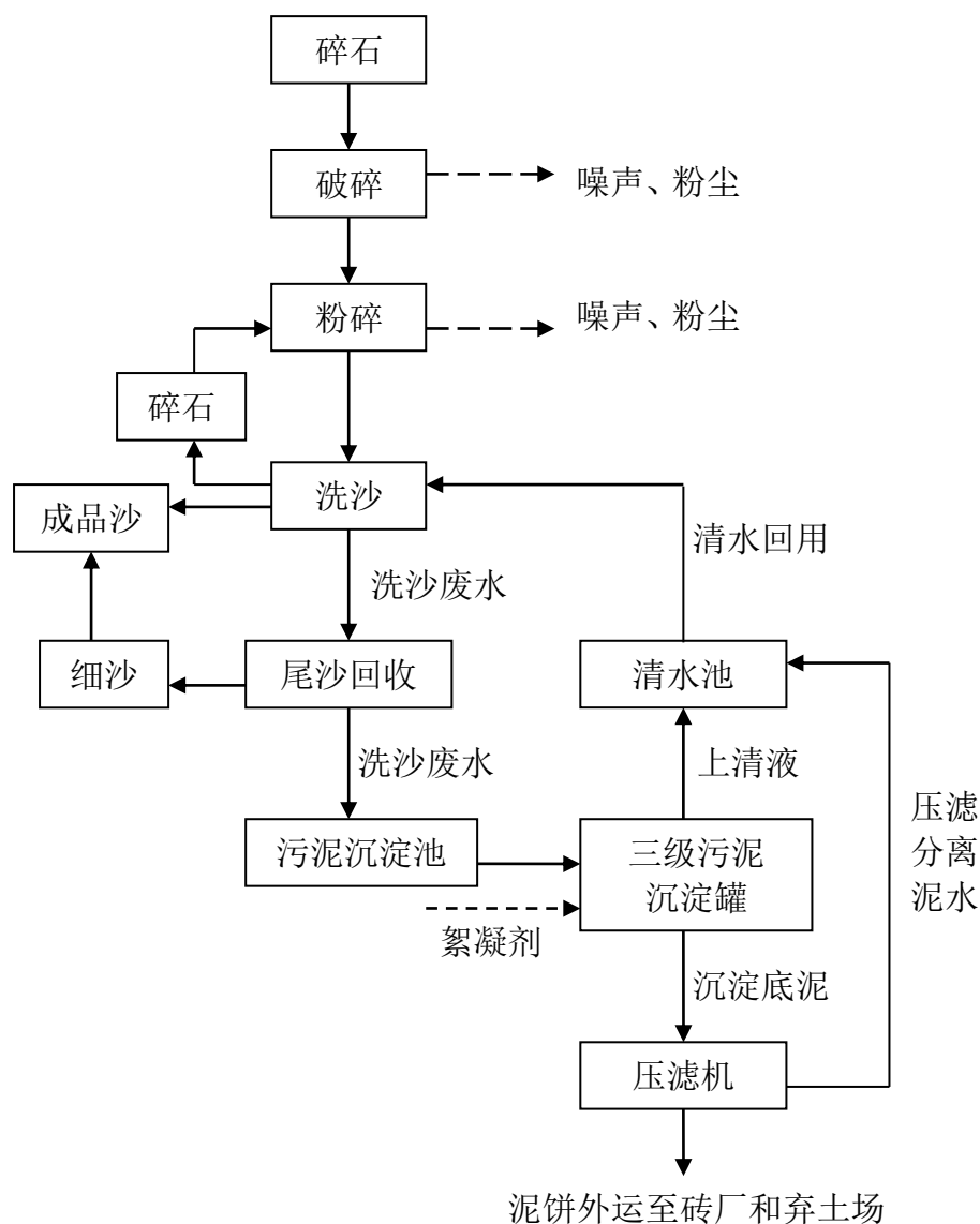
图 2-2 项目生产工艺流程及产污环节图
